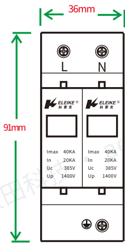
前视图
